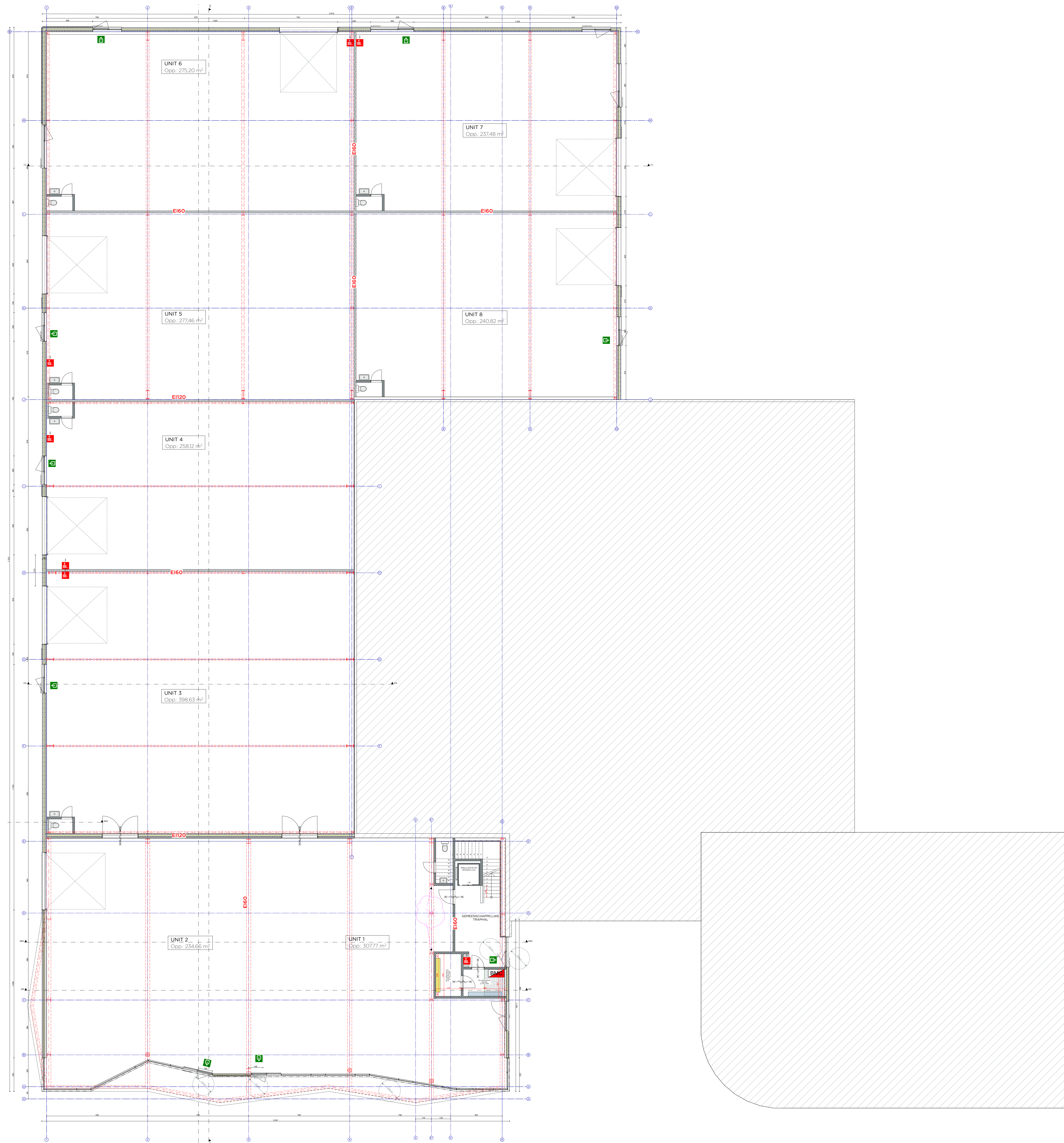
S:1:100 Gelijkvloers
